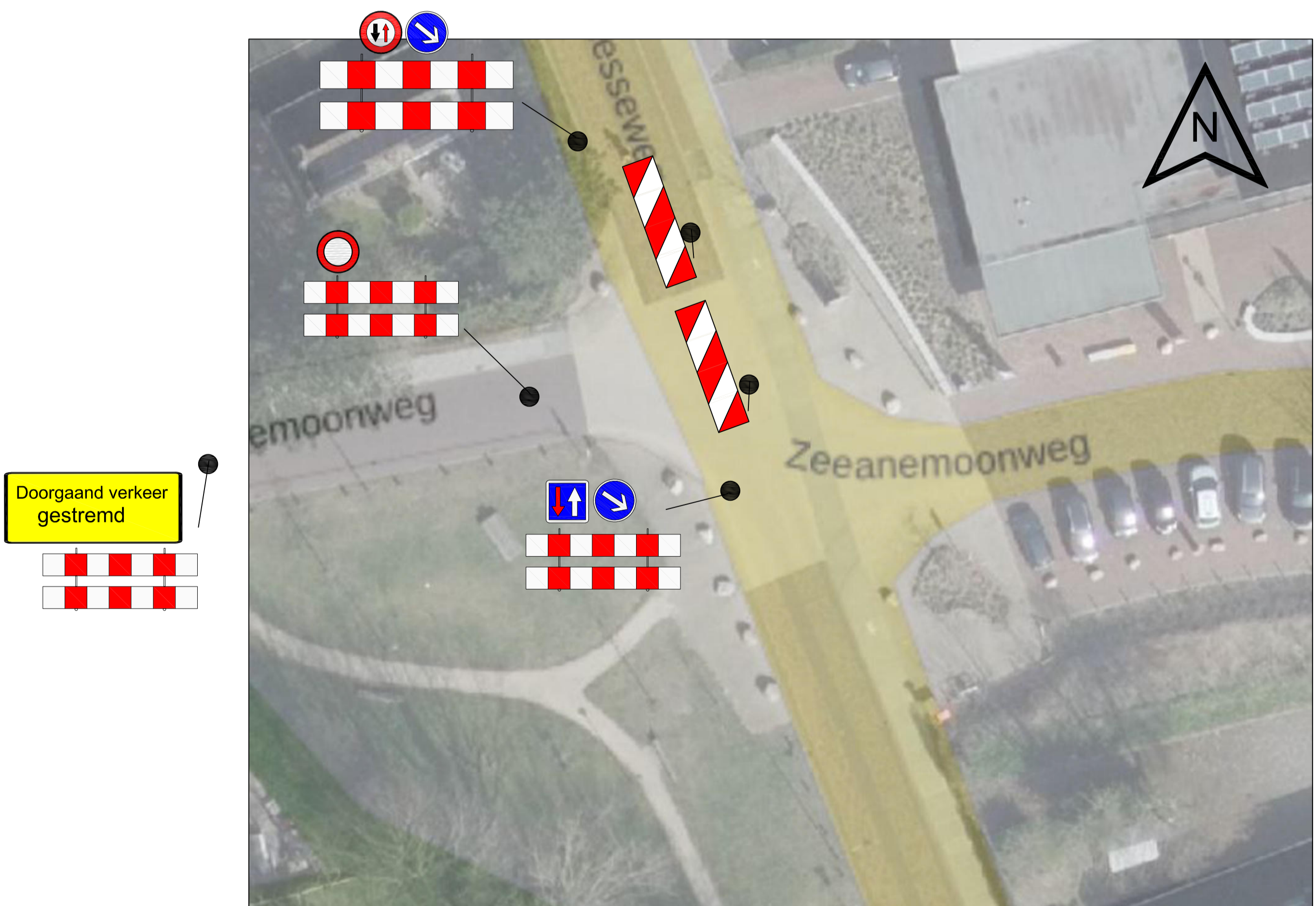
Fase 2: met vooraankondiging werk in Uitvoering en snelheidsbeperking 30km/h
