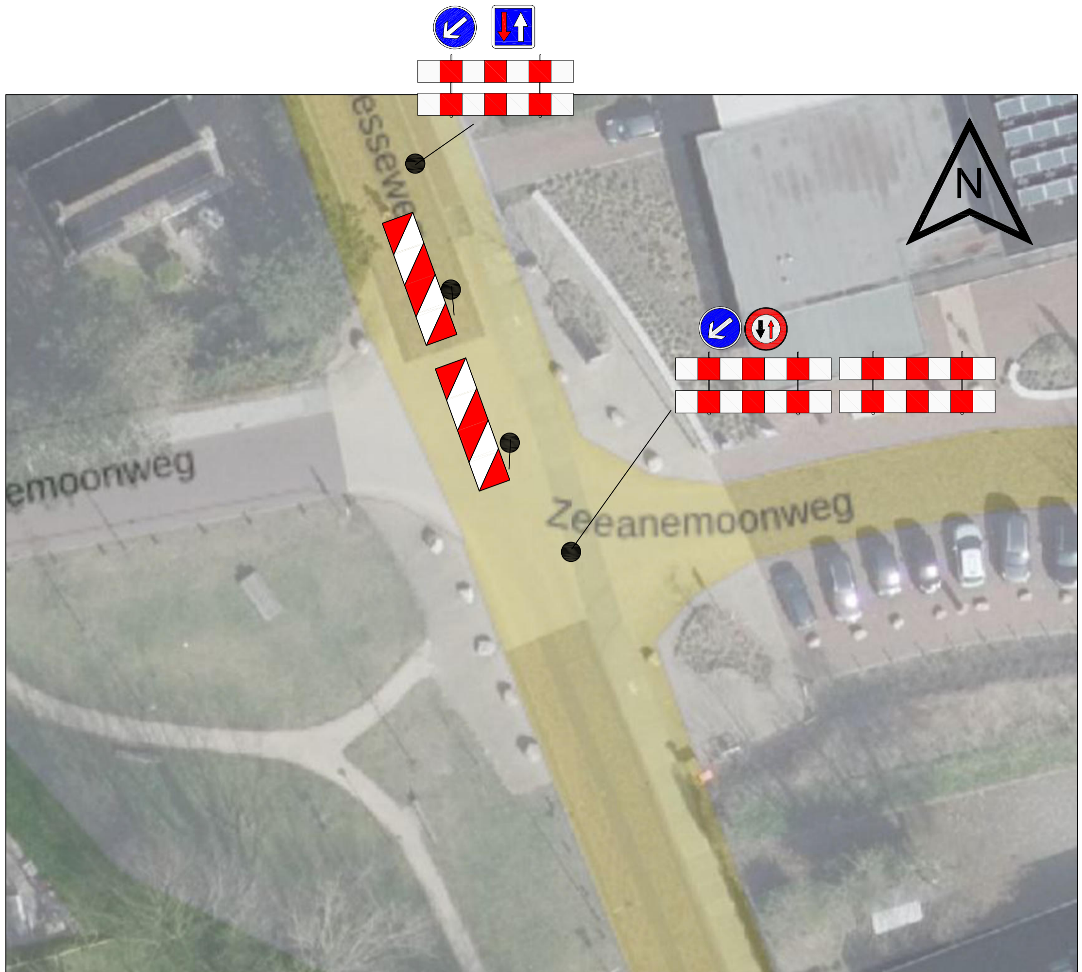
Fase 1: met vooraankondiging werk in Uitvoering en snelheidsbeperking 30km/h
